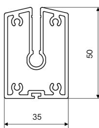
ALAPROFIIL BD 50
