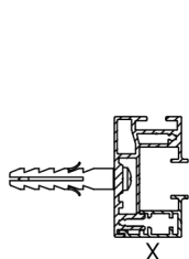
KÜLJELE PAIGALDAMINE
