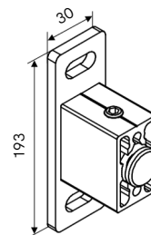
F-KINNITUS
