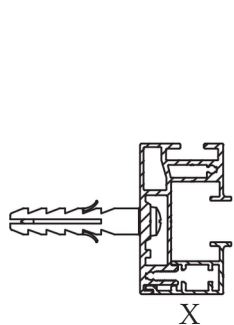
KÜLJELE PAIGALDAMINE
