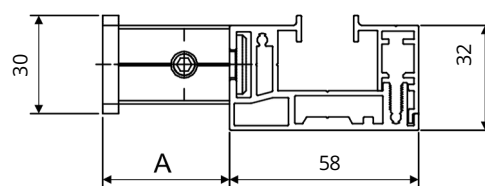
GS 35 KÜLGSIIN F-KINNITUSEGA
