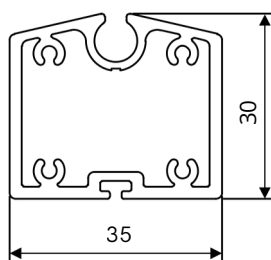
ALAPROFIIL BD 30
