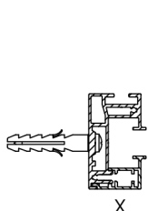
KÜLJELE PAIGALDAMINE
