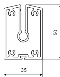
ALAPROFIIL BD 50
