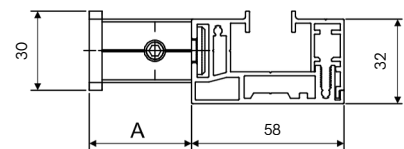
GS 35 KÜLGSIIN F-KINNITUSEGA
