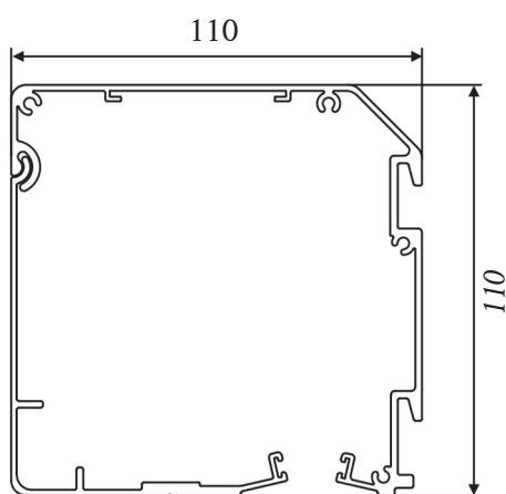
KASSETT 110
