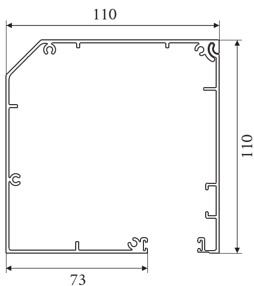
KASSETT 110
