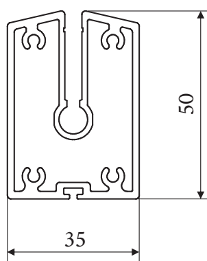
ALAPROFIIL BD 50
