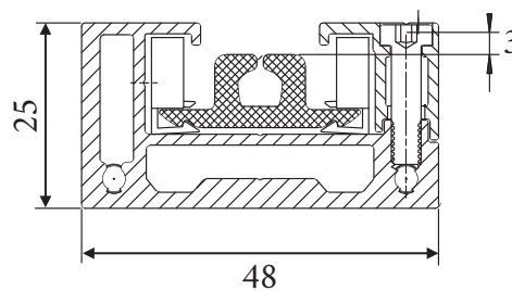
GS 25 KÜLGSIIN
